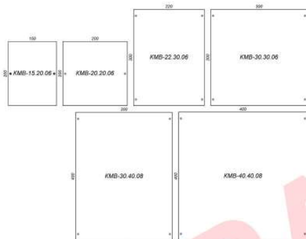
Рис.2 Внешний вид коробок серии KMB
