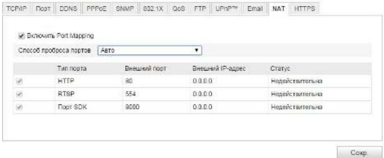
Рисунок 6-15 Настройка NAT
