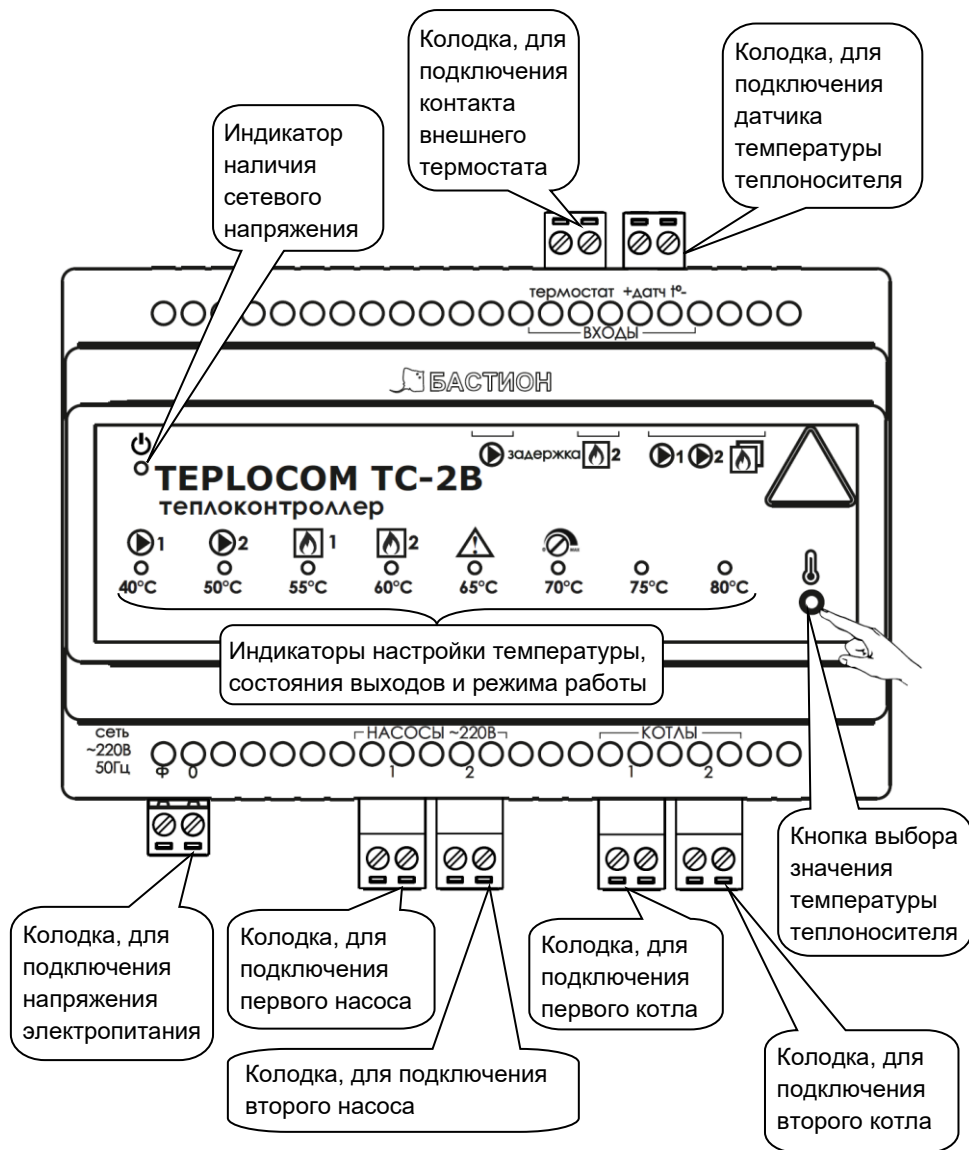
Рисунок 2 — Общий вид передней панели изделия
