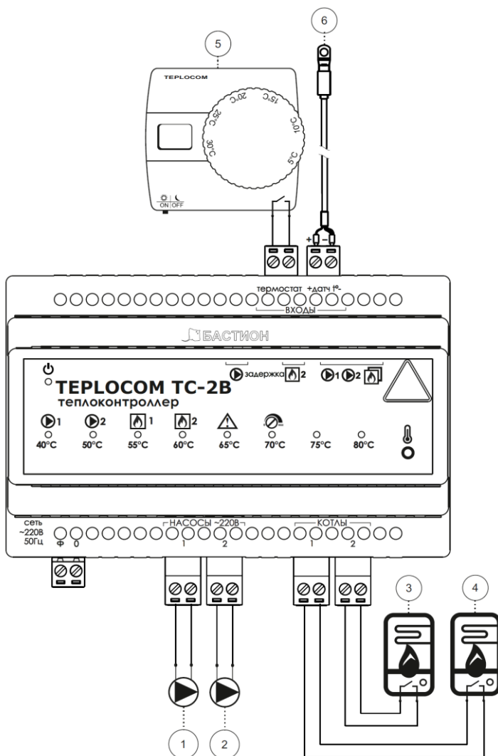
Рисунок 5 – Схема подключений
