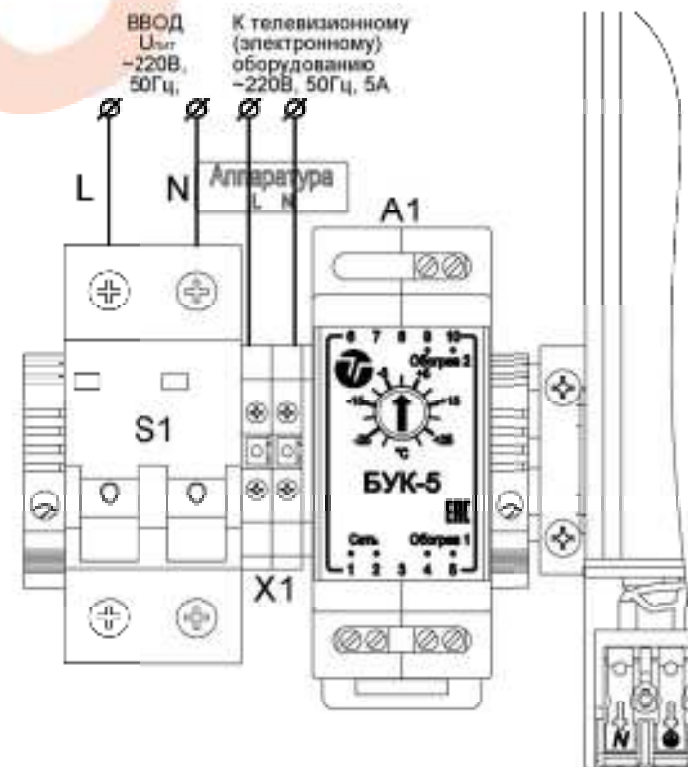
Рис.2. Подключение термощафа
