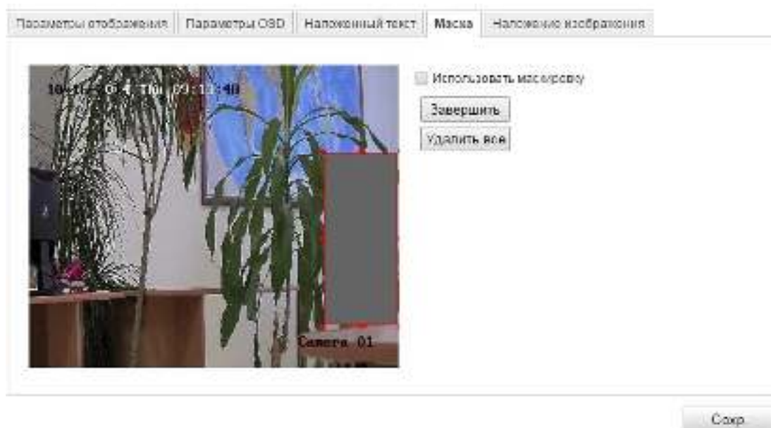
Рисунок 6-31 Настройки маски
