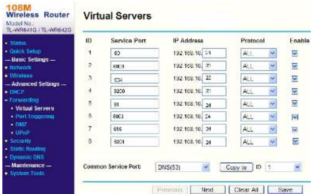
Рисунок П-2.3 Конфигурация портов
