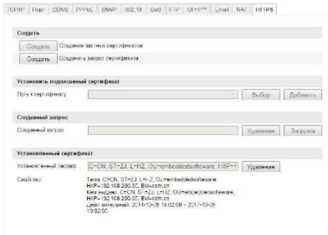
Рисунок 6-17 HTTPS настройки
